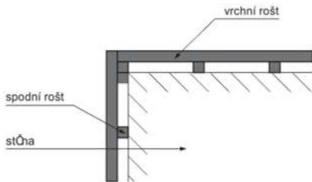
Ukázka rohového uchycení roštu
